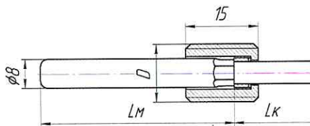
Рисунок 2 – Эскиз датчиков конструкции 2
