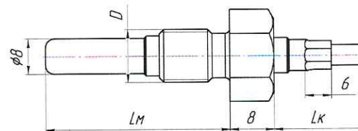
Рисунок 4 – Эскиз датчиков конструкции 4
