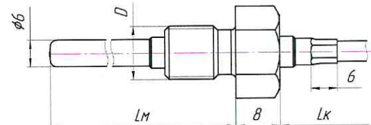
Рисунок 3 – Эскиз датчиков конструкции 3
