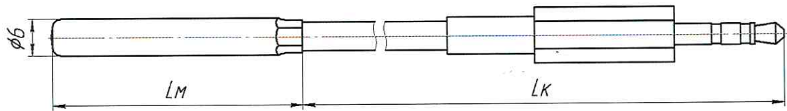
Рисунок 1 – Эскиз датчиков конструкции 1
